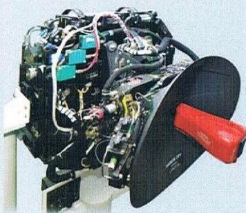
Das Bordradar NASARR des F-104 'Starfighters' wurde zu Beginn der 70er Jahre in Ulm in Serie gefertigt
